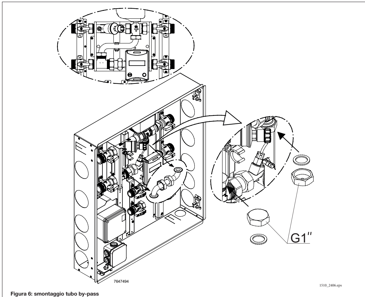
Figura 6: smontaggio tubo by-pass
