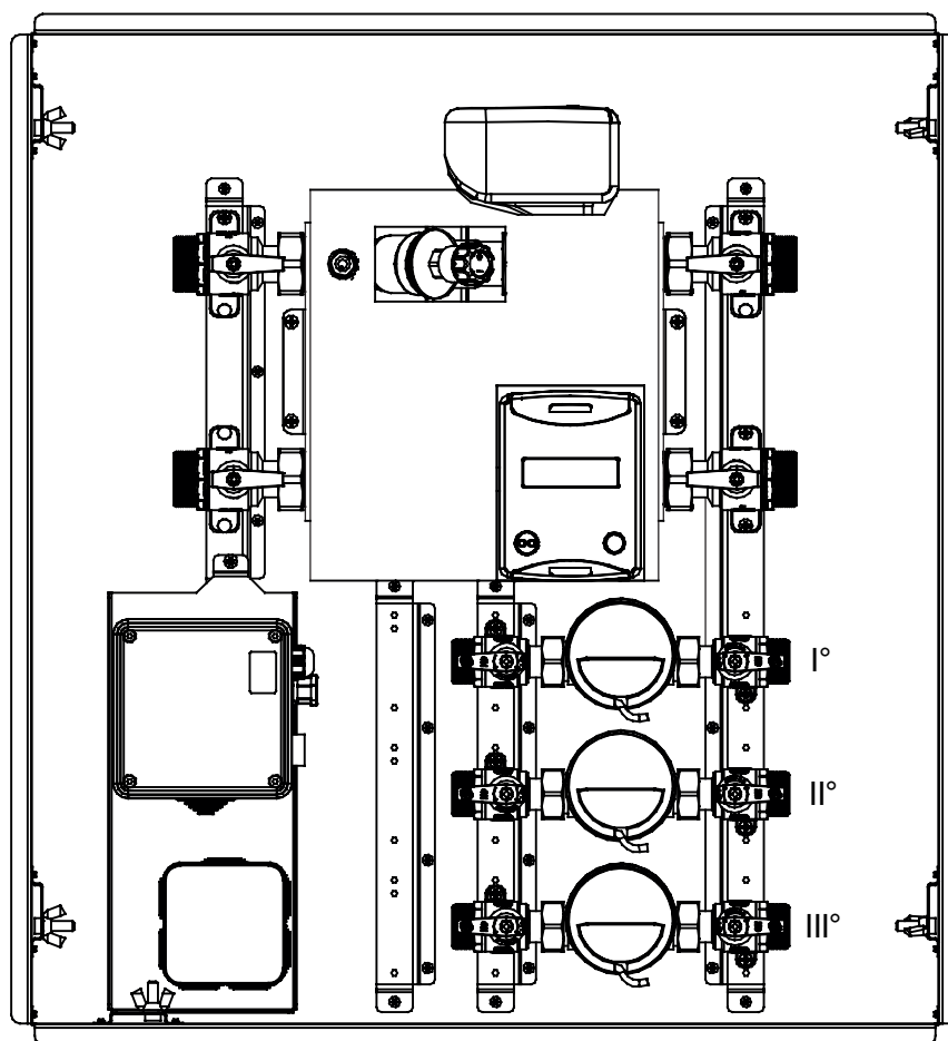
Figura 8A: Contatori consumo acqua sanitaria
