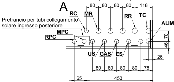
INSTALLAZIONE POSTERIORE (vista frontale)
