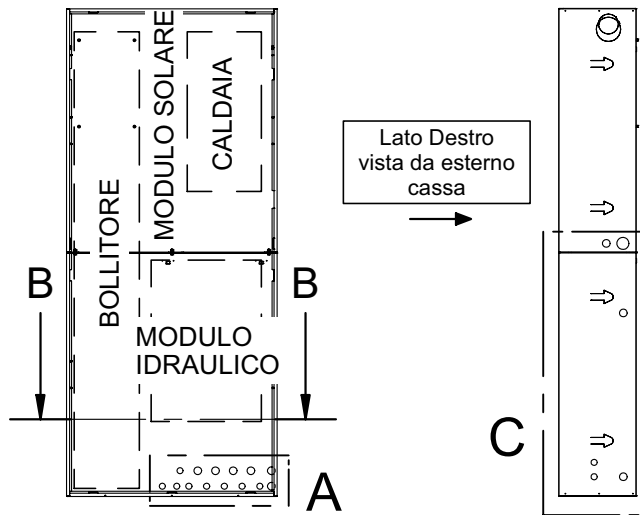
INSTALLAZIONE POSTERIORE (vista frontale)
