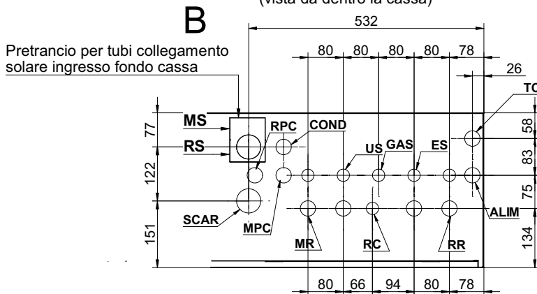
INSTALLAZIONE INFERIORE (vista da dentro la cassa)
