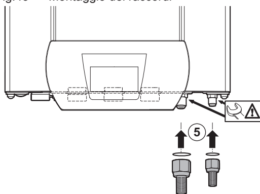
Fig.43 Montaggio dei raccordi
