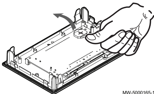
Fig.123 Rimuovere la batteria
