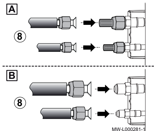
Fig.45 Collegamento dei tubi
