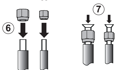
Fig.44 Montaggio dei dadi
