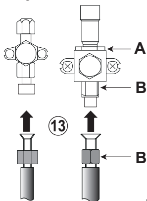
Fig.48 Collegamento dei tubi
