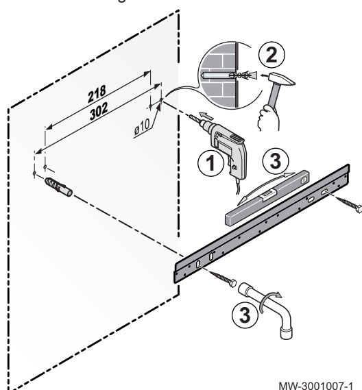
Fig.29 Realizzazione dei fori e montaggio della guida
