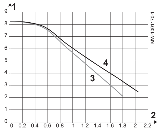
Fig.3 Pressione disponibile
