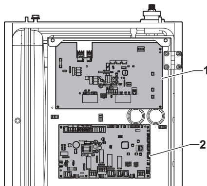
Fig.15 Ubicazione delle schede elettroniche
