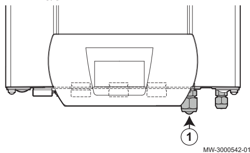
Fig.39 Allentamento parziale del dado da 5/8"
