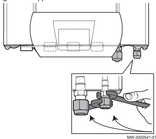
Fig.39 Allentamento parziale del dado da 5/8"
