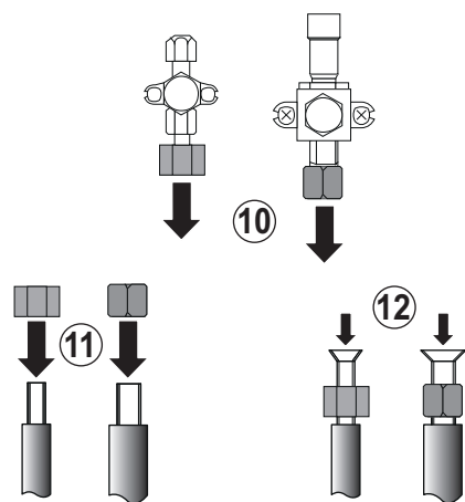
Fig.47 Svitare i dadi delle valvole di isolamento
