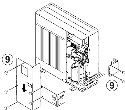
Fig.46 Rimozione dei pannelli laterali
