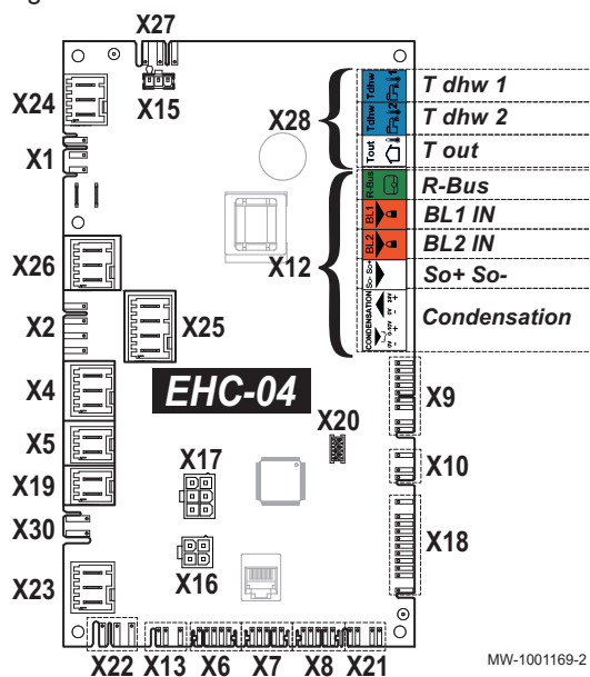
Fig.53 Morsetteria del modulo interno
