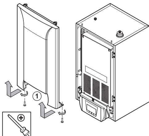
Fig.36 Rimozione del pannello anteriore
