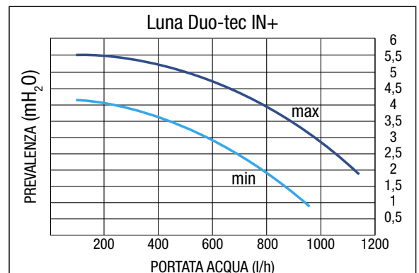
Grafico pompa
