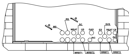
INSTALLAZIONE POSTERIORE (vista frontale dentro la cassa)
