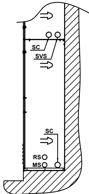
VISTA LATO DESTRO (vista da esterno cassa)
