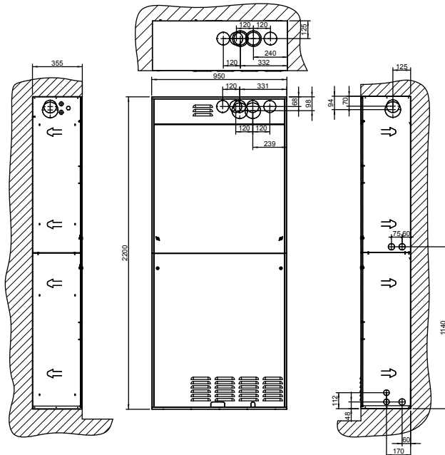
Dima di montaggio
