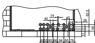
INSTALLAZIONE POSTERIORE (vista frontale dentro la cassa)
