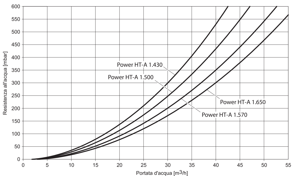
Fig. 2: Diagramma della resistenza sul lato acqua Power HT-A 1.430-1.650
