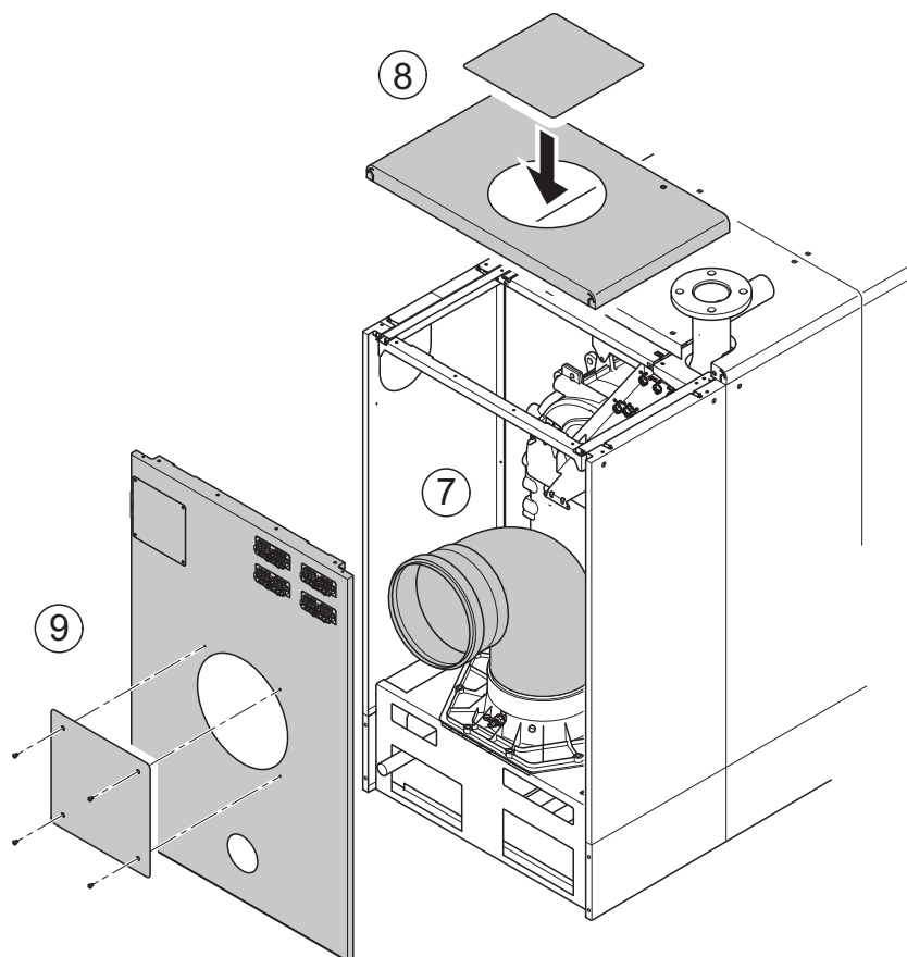
Fig. 24: Montaggio della curva da 87°(accessorio)
