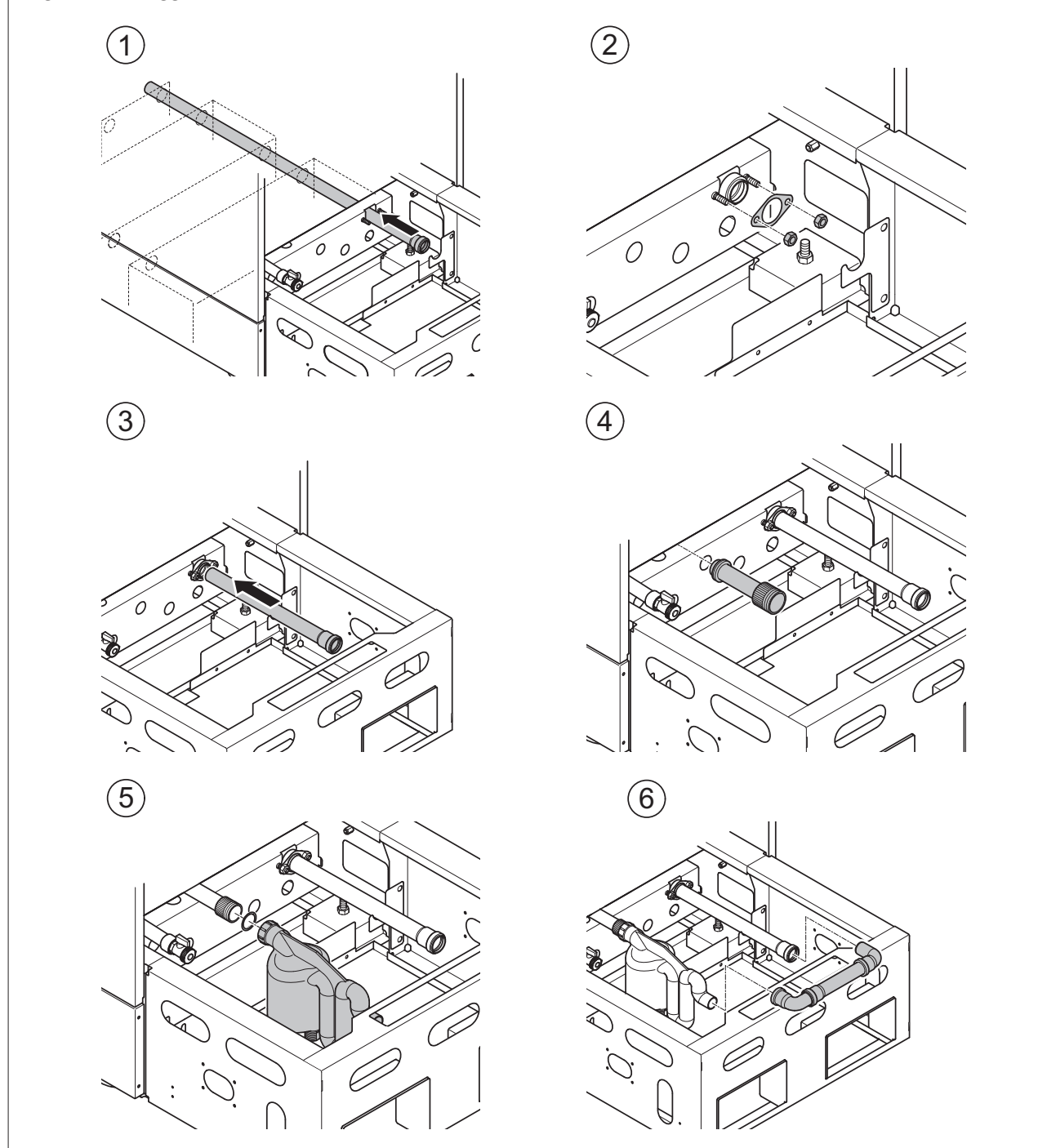
Fig. 18: Montaggio del sifone e dei tubi della condensa
