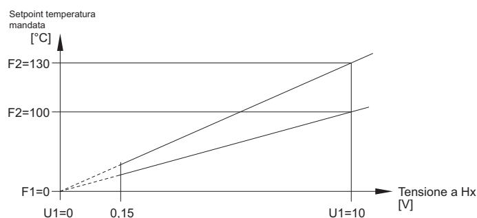
Fig. 48: Esempio per richiesta termica 10 V e richiesta freddo 10 V
