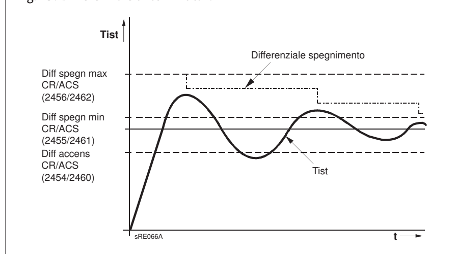
Fig. 43: Differenziale di commutaz.
