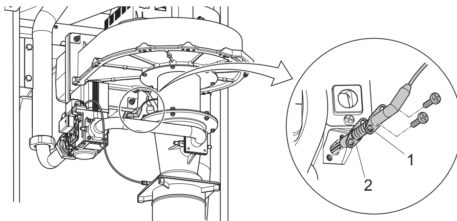
Fig. 54: Sostituzione dell'elettrodo di accensione e ionizzazione
