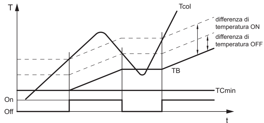
Fig. 44: Regolazione carico /schematico)
