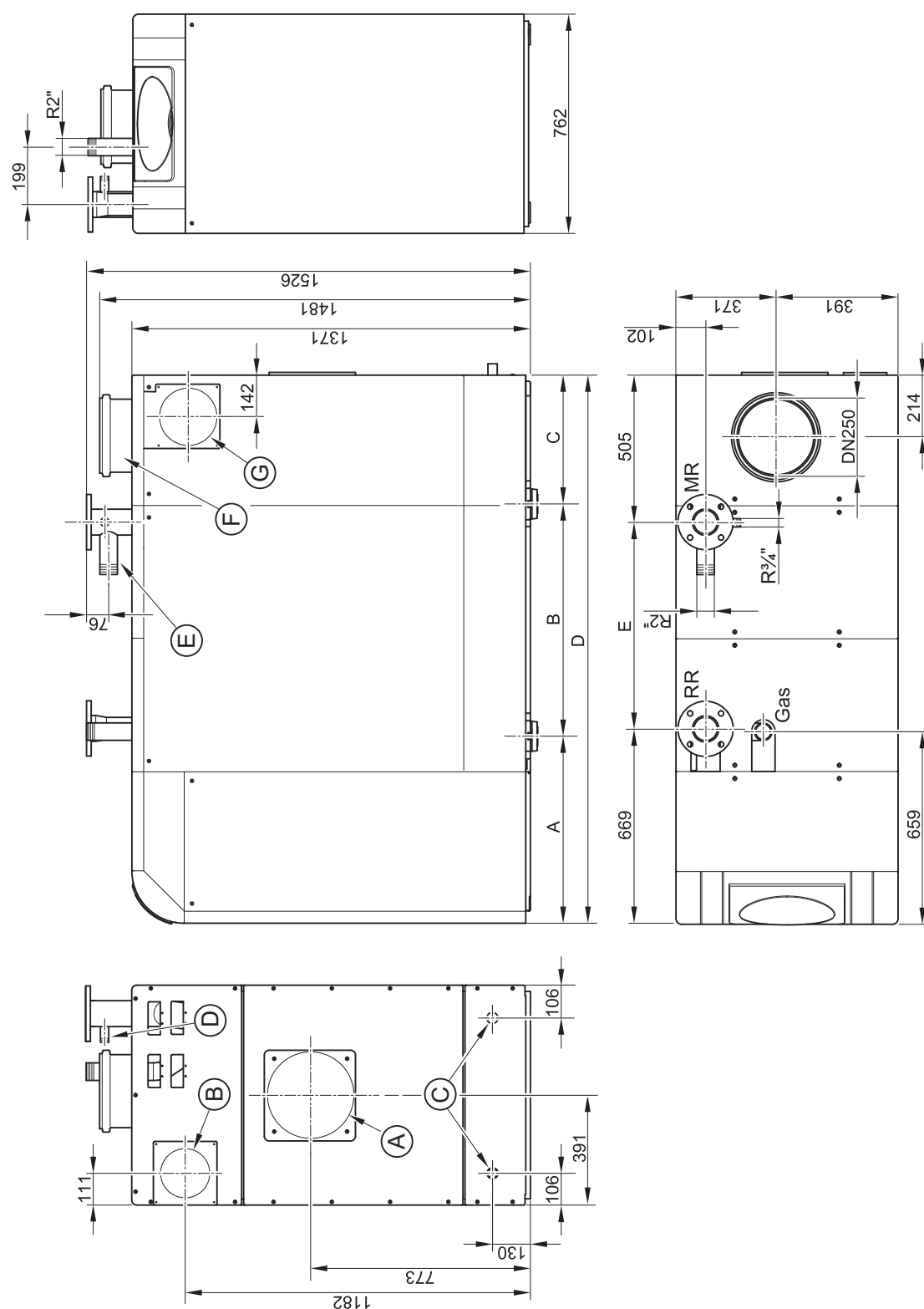
Fig. 1: Dimensioni ed attacchi
