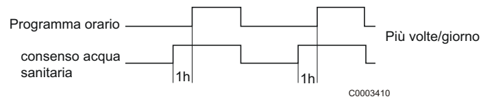
Fig. 46: Anticipo carico
