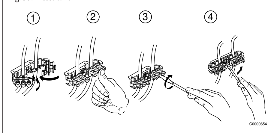
Fig. 30: Pressacavo
