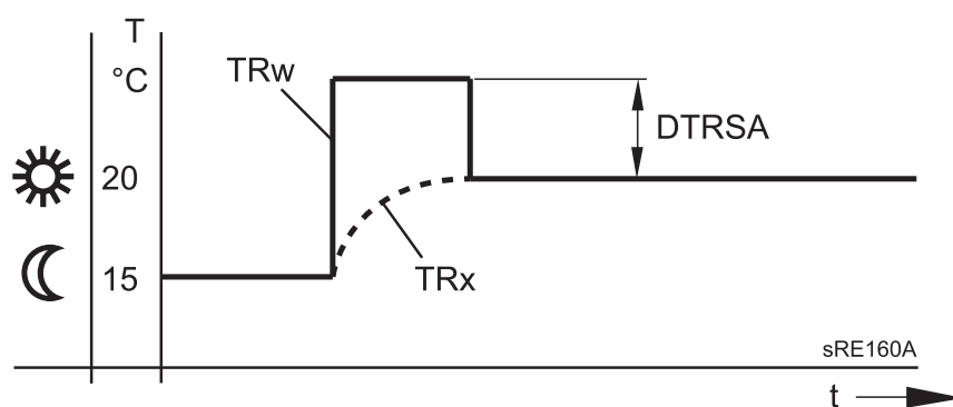
Fig. 37: Riscaldamento accelerato
