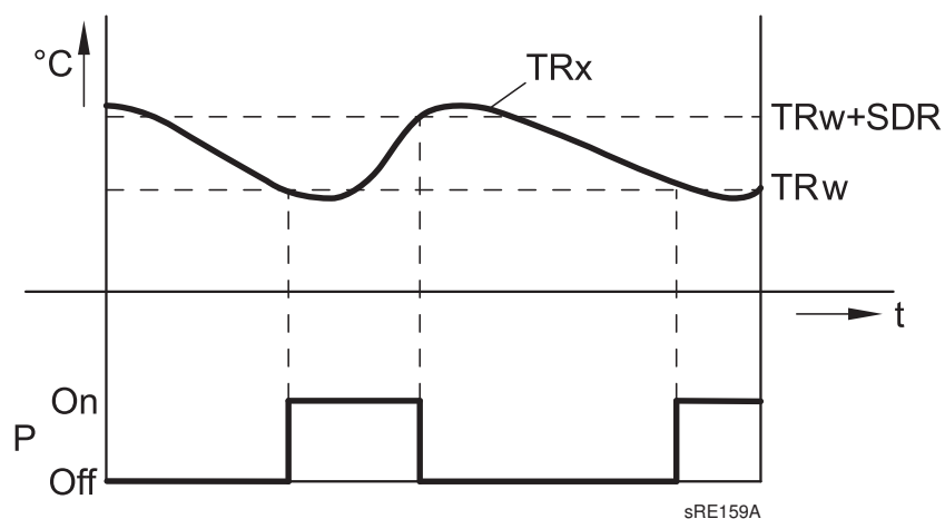
Fig. 36: Limitazione temp. ambiente
