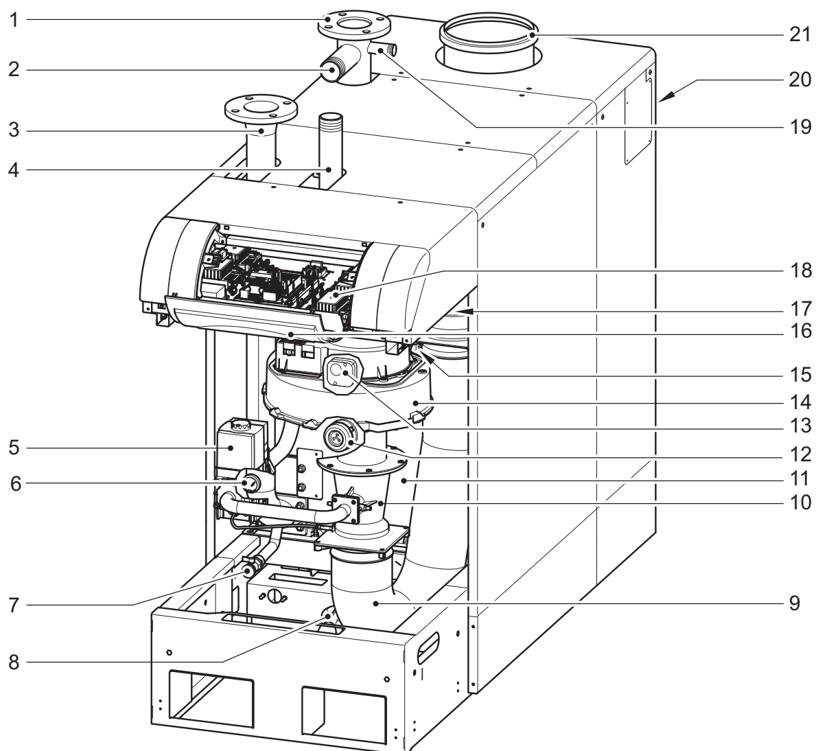
Fig. 50: Vista caldaia Power HT-A 1.650
