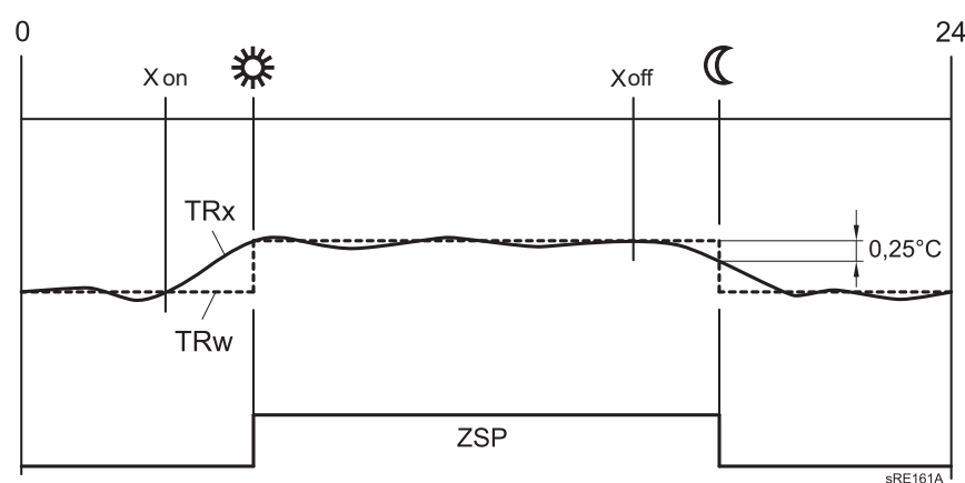
Fig. 38: Ottimizzazione all'accensione ed allo spegnimento
