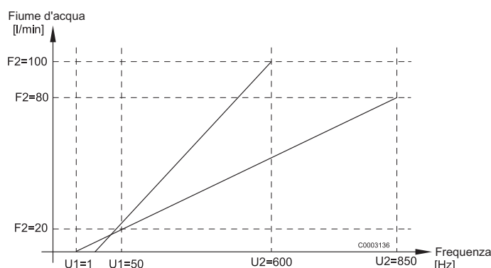
Fig. 47: Esempio per due differenti curve caratteristiche della sonda
