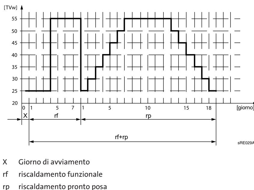
Fig. 40: Profilo di temperatura nella funzione asciugatura massetto
