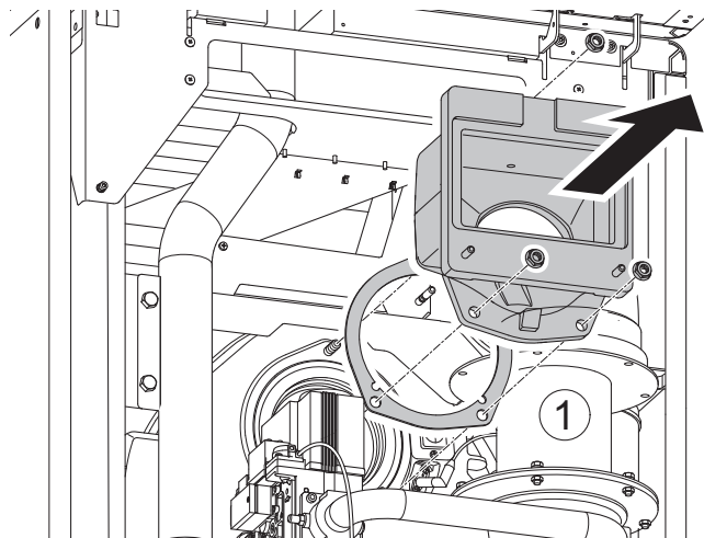
Fig. 56: Rimuovere l'adattatore del miscelatore
