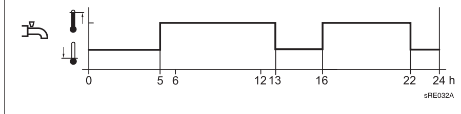
Fig. 42: Via libera in base al programma orario 4 (esempio)
