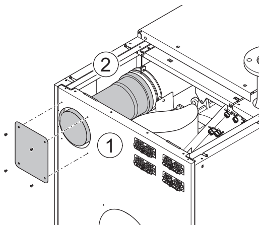
Fig. 25: Montaggio degli attacchi dell'adduzione dell'aria
