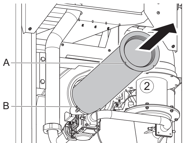
Fig. 57: Rimuovere il bocaglio del bruciatore
