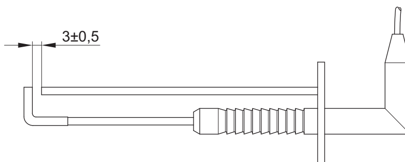
Fig. 55: Distanza dell'elettrodo
