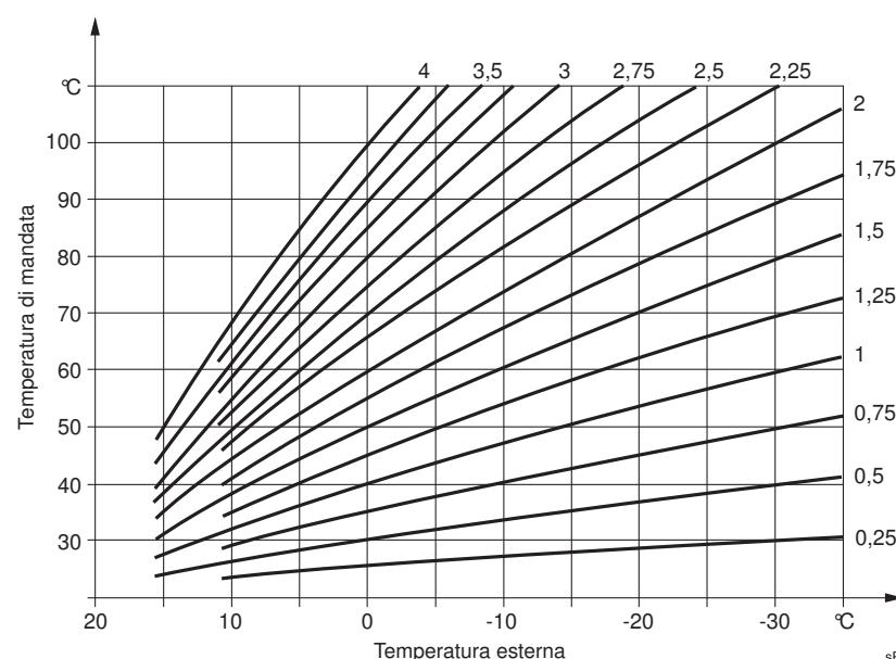
Fig. 34: Diagramma curve caratteristiche riscaldamento
