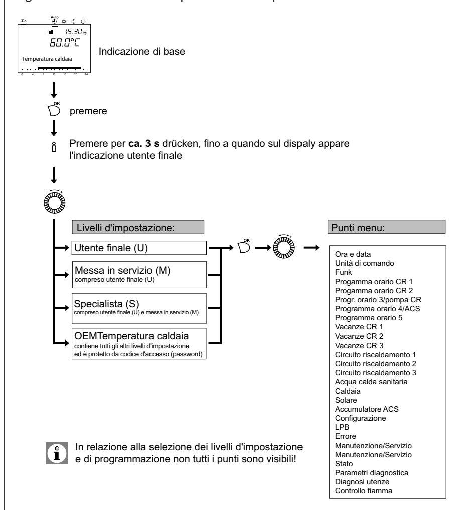
Fig. 33: Selezione dei livelli impostazione e dei punti menu
