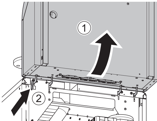
Fig. 9: Sollevamento della cassetta di regolazione
