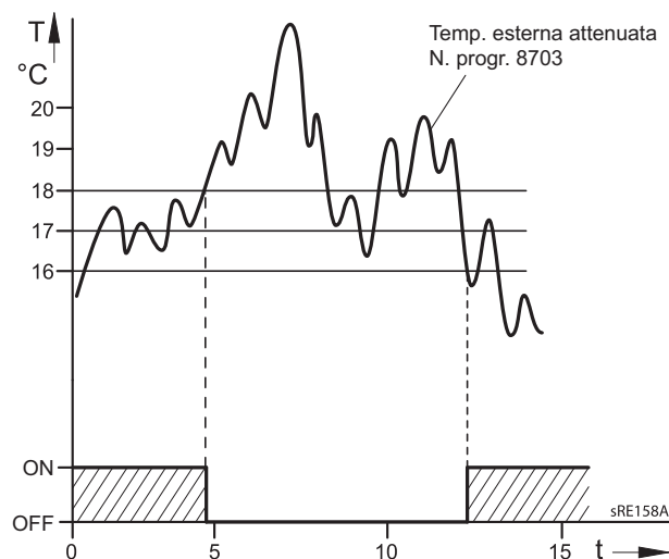
Fig. 35: Valore limite estate/inverno
