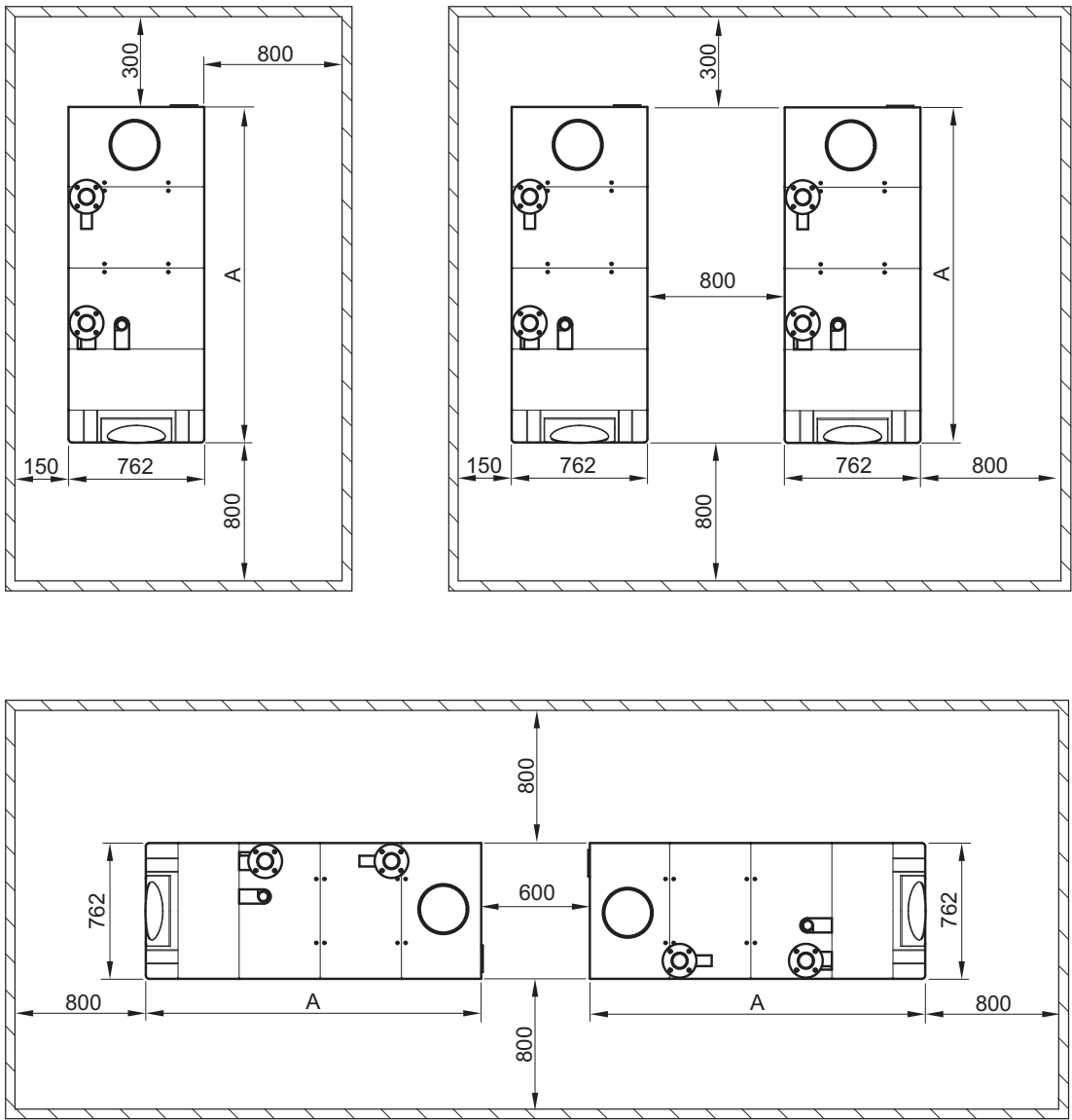
Fig. 4: Ingombro consigliato
